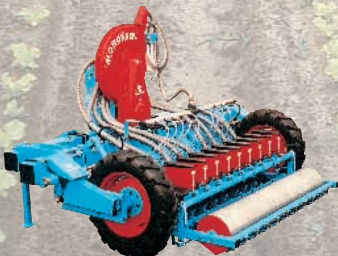
MS E : Sembradora minigranos para sembrar en mesas
